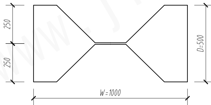
俯视图 1:15
