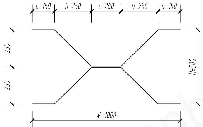
主视图 1:15
